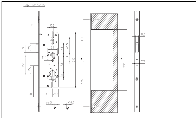
Abb. 6 Hauptschloss RGS RS1000SL für Dornmaß 55 und 65, Entfernung 72 mm
