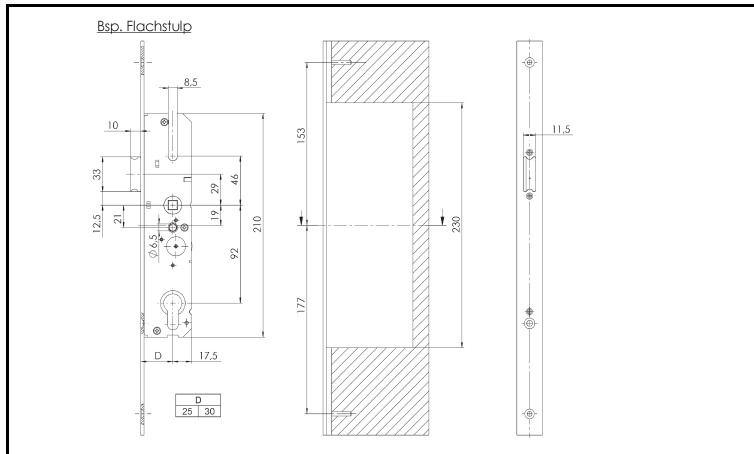
Abb. 7 Hauptschloss RGS RS1000SL für Dornmaß 35 - 65, Entfernung 92 mm
